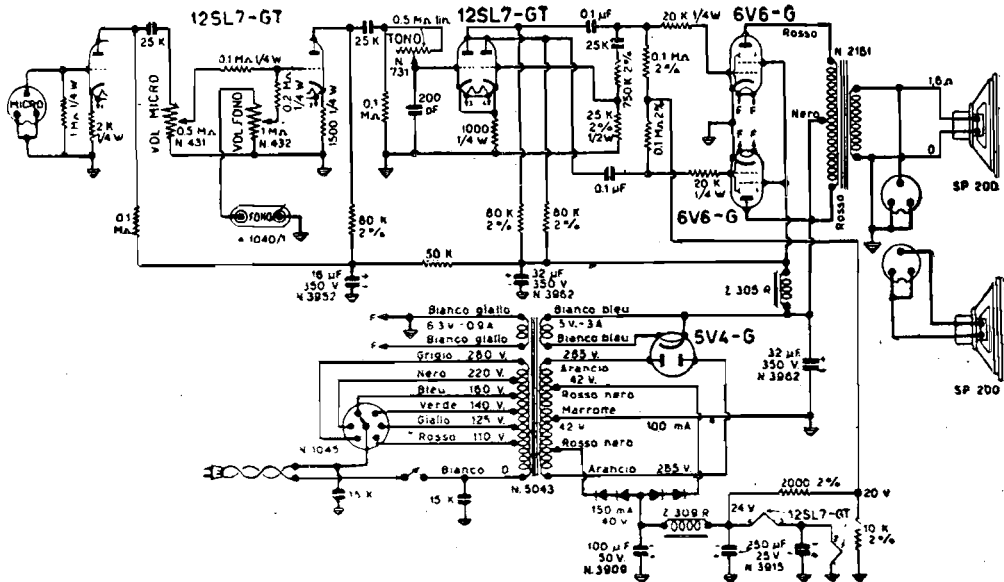
GELOSO - Amplificatori portatili a valigia modd. G-250/V e G-213/V. Potenza 12 watt con 5% di distorsione. Lo schema è quello del mod. G-205/V, il mod. G-213/V differisce per avere il trasformatore d'uscita con prese al secondario.
